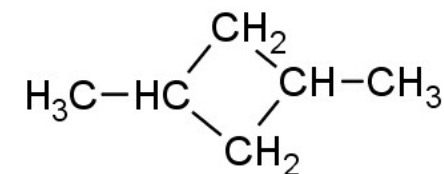
1,3-dimethylcyklobutan
