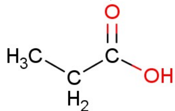
Propansyre
